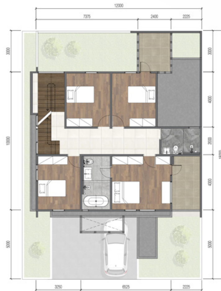
Lantai 2
